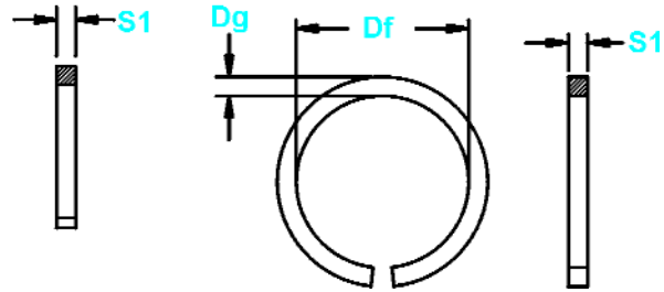
Durchmesser im ungespannten Zustand und Ringabmessung mit Schnitt B-B
