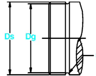
Wellendurchmesser & Nutabmessungen
